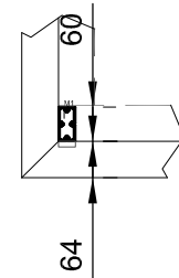
Mitred Corner Horizontal Section
