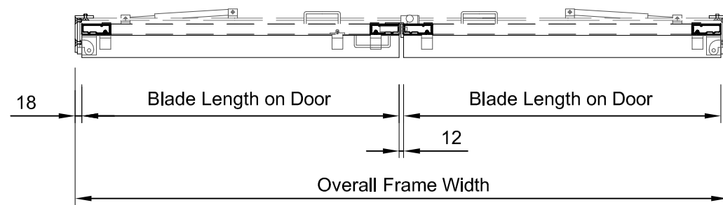
Double Door Horizontal Section
