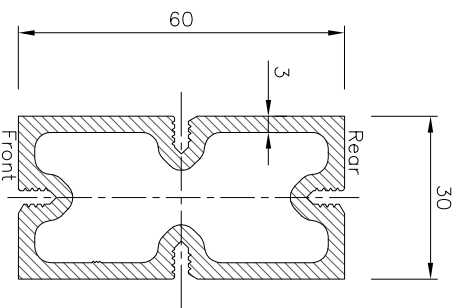
M1 Mullion
