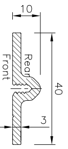
M3 Mullion
