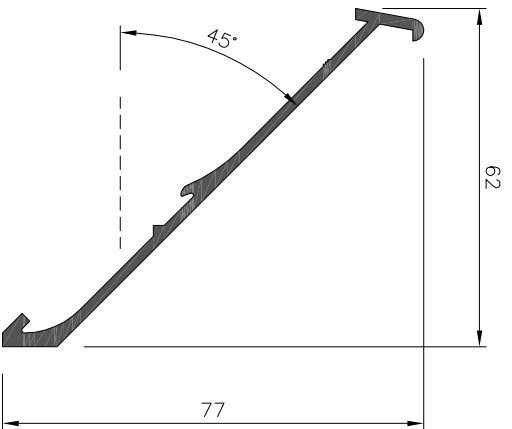
KW50Z Blade
